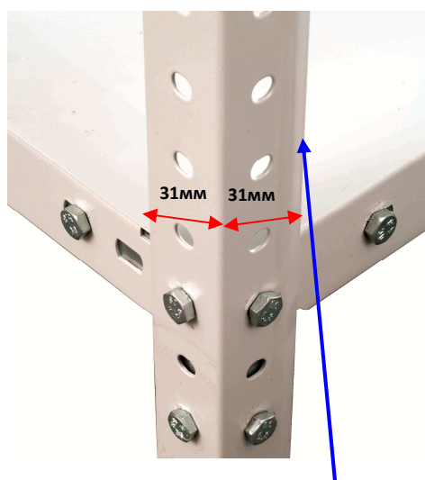
Профилированный усиливающий элемент
