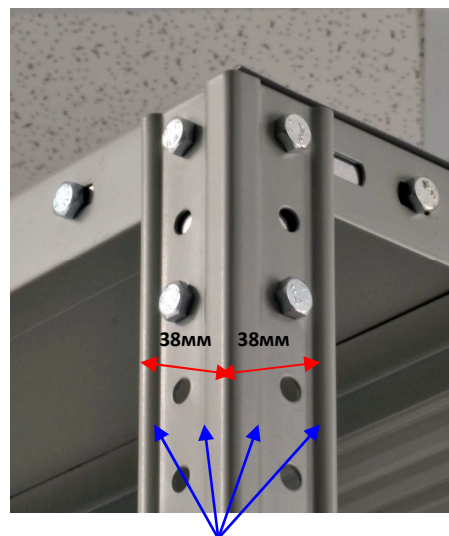
Профилированные усиливающие элементы
