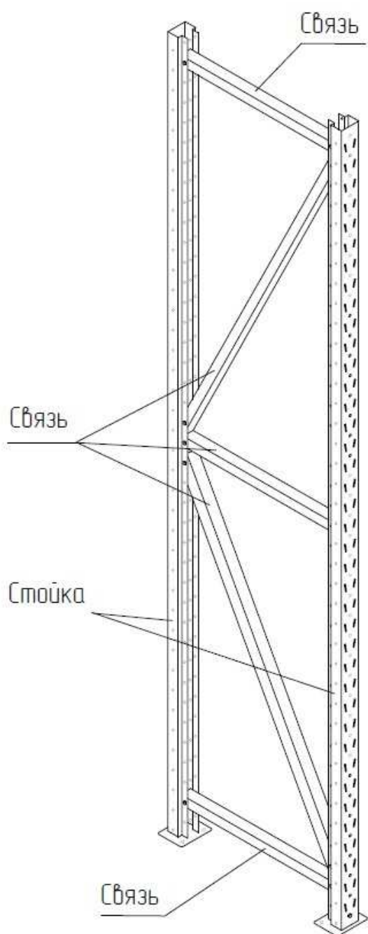
Рис. 1. Рама в сборе.
