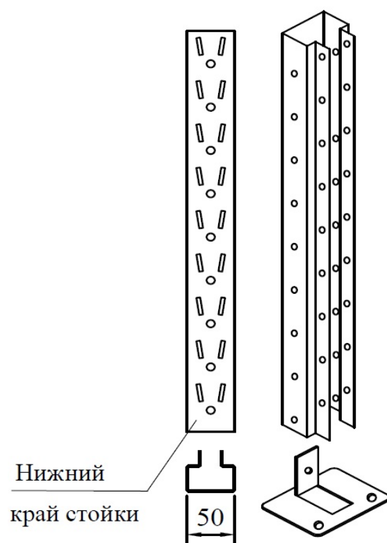
Рис. 2. Стойка.
