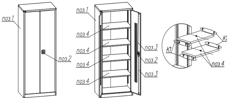
Рис. 2 Устройство архивных шкафов сери WA
